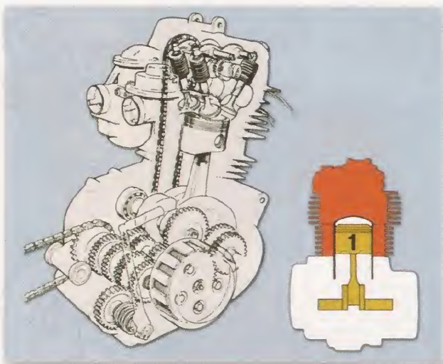
Motor monocilíndrico
